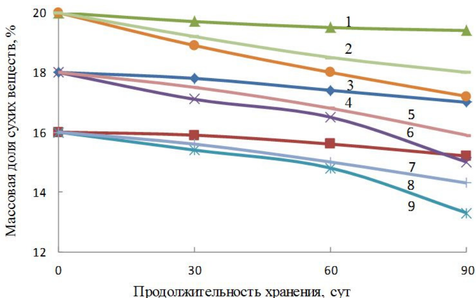
Рисунок 2. – График изменения массовой доли сухих веществ мармеладных изделий в процессе хранения: 1, 4, 7 – в металлизированной пленке; 2, 5, 8 – в полиэтиленовой стрейч-пленке; 3, 6, 9 – в открытой таре.
